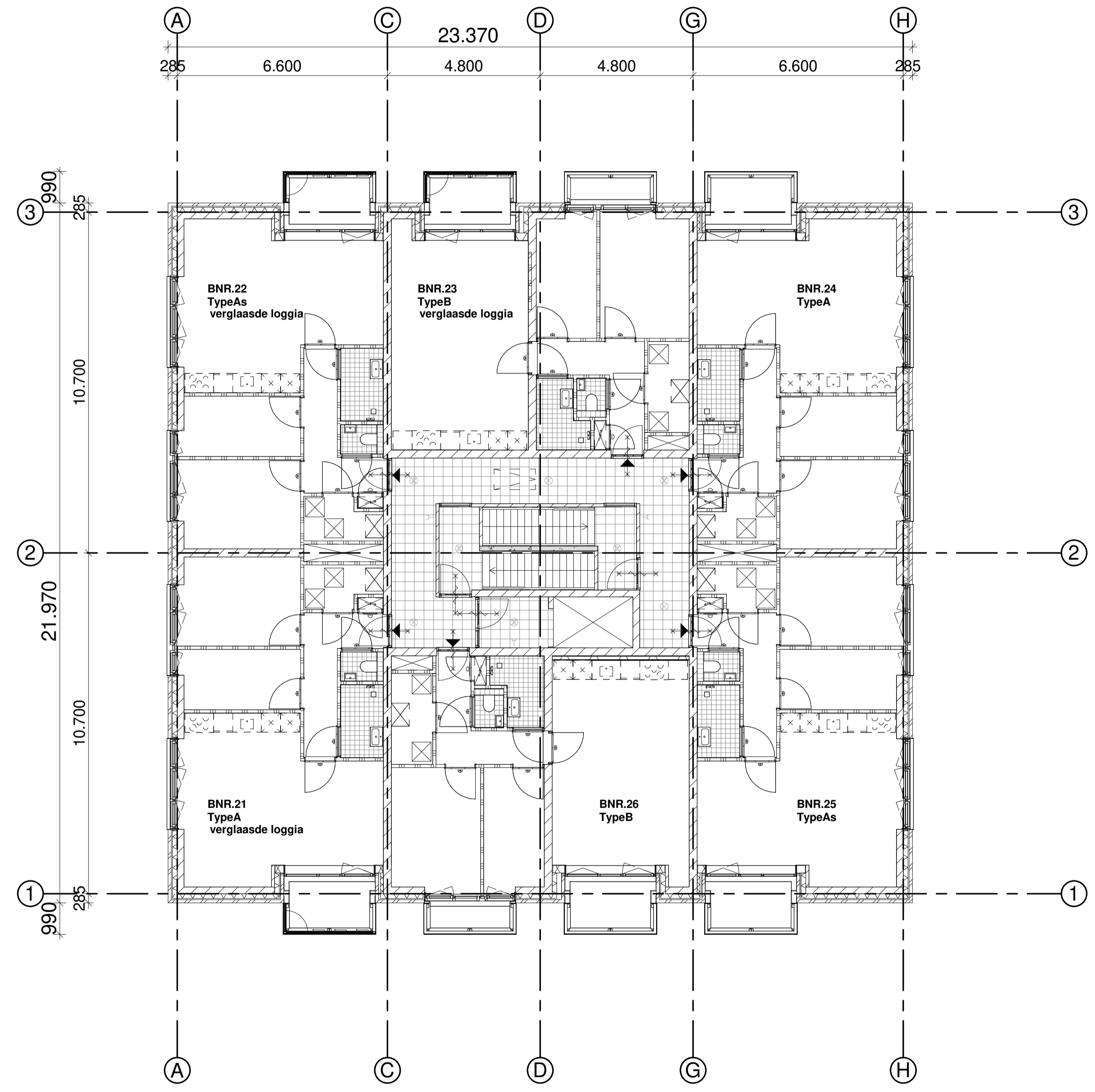
plattengrond vierde verdieping 1:100
