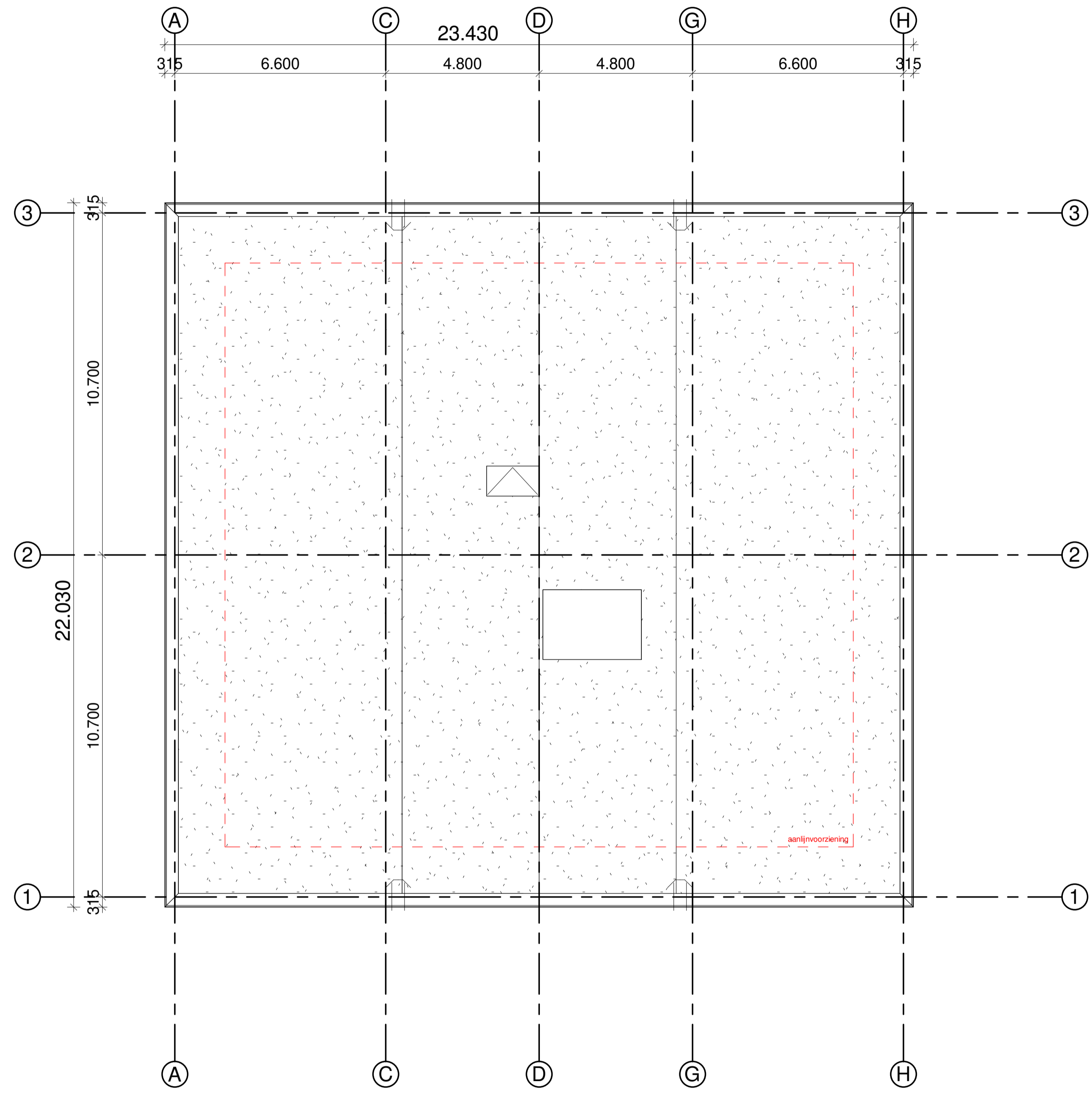
plattengrond dak 1:100
